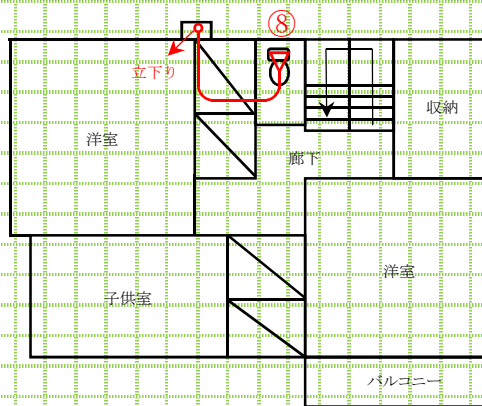
2階平面図
