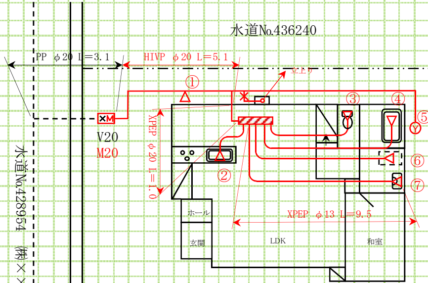
1階平面図
